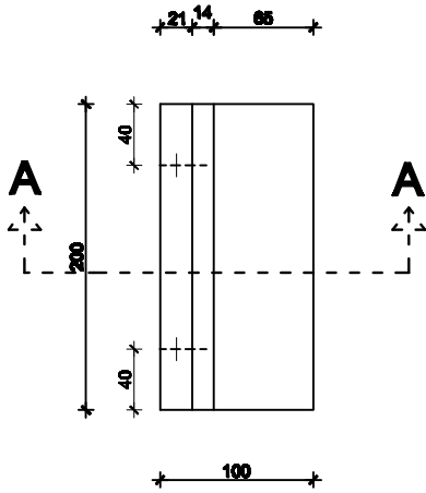
tlocrt
