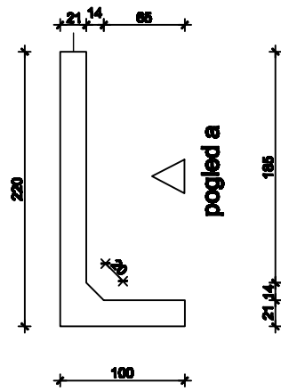
presjek A-A
